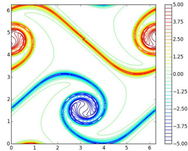
(d) Vorticity at t = 7 , Algorithm 5
