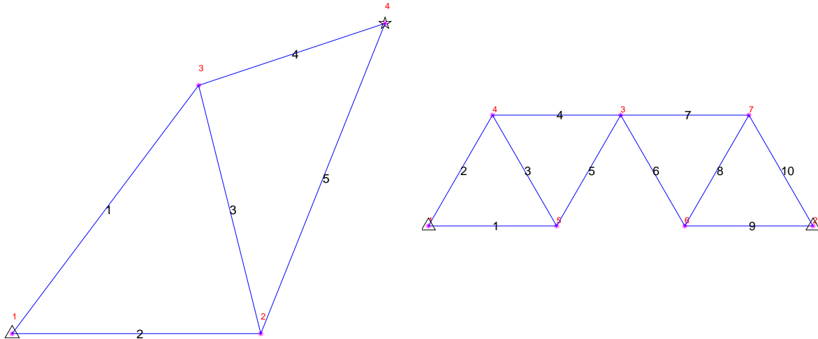
Abbildung 1: Beispiel für die Visualisierung von Fachwerken. Das linke Fachwerk entspricht dem Beispiel aus Abschnitt 5.5.1 der Vorlesung, das rechte dem Fachwerk aus Figure 11.6 aus dem Buch “Ingenieurmechanik I” von Sayir, Dual und Kaufmann (Vieweg/Teubner 2008). Gelenke sind durch * in der Farbe Magenta bezeichnet, Stäbe durch blaue Linien, Auflager durch schwarze Pentagramme und feste Lager durch schwarze Dreiecke.
